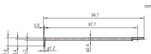
Щуп для измерения волнистости [двойной длины]
