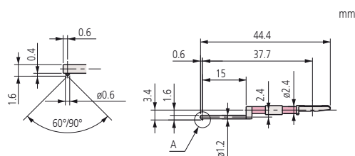
Щуп для малых отверстий
