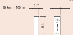
Номинальная длина: 10.3 мм - 100 мм
