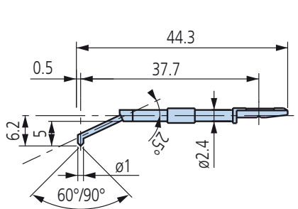
Щуп для дна глухого отверстия
