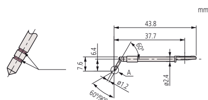
Щуп для зубьев шестерен
