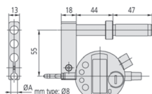
12AAA792 (с опциональным индикатором)
