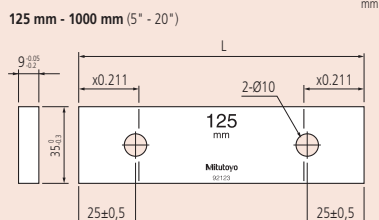
Номинальная длина: 125 мм - 1000 мм
