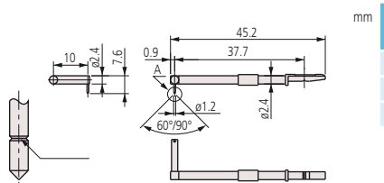
Щуп для эксцентриковой консоли
