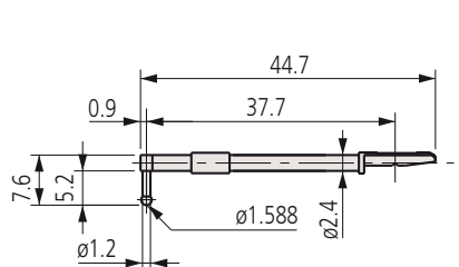
Щуп для глубоких канавок 40 мм
