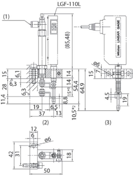
Для датчика линейных перемещений с диапазоном измерений 10 мм LGF-125L / LGF-150L
