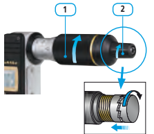
1 : Трещотка на барабане 2 : Трещотка на ускорителе
