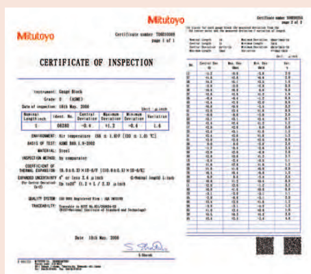
Концевые меры и сертификат контроля Mitutoyo
