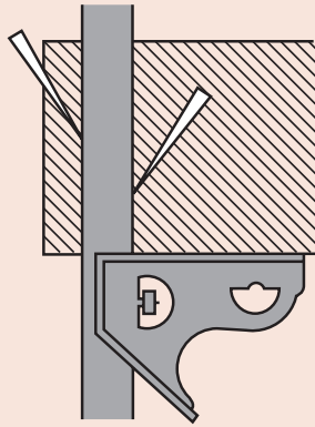
180-102B Прямоугольная головка
