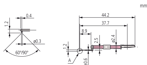
Щуп для малых отверстий
