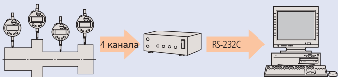
Интерфейс MUX-10F
