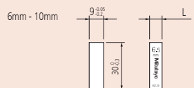
Номинальная длина: 6 мм - 10 мм
