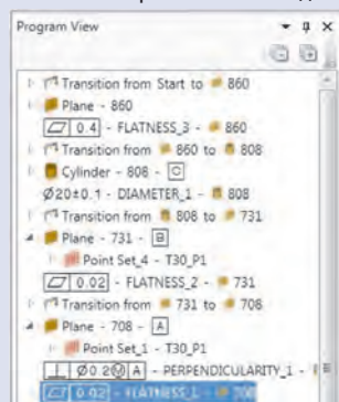
Шаг 4: Создайте программу измерения
