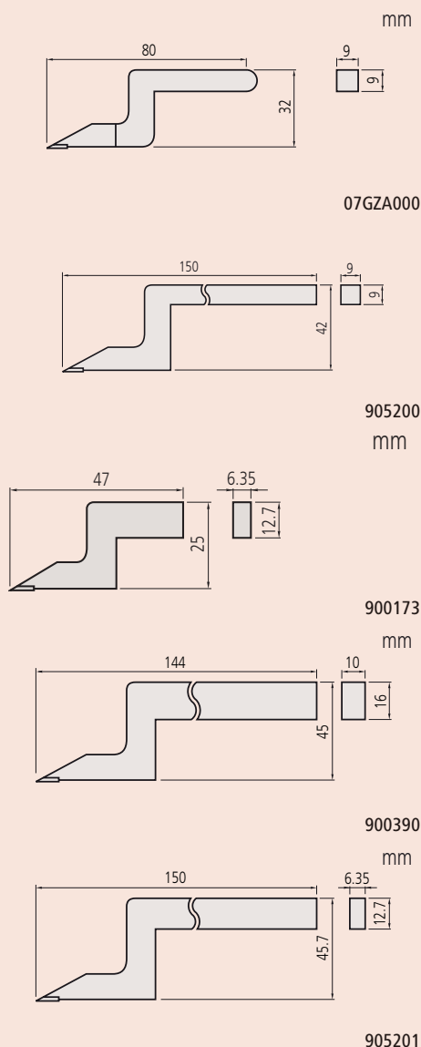
Твердосплавные разметочные ножки
