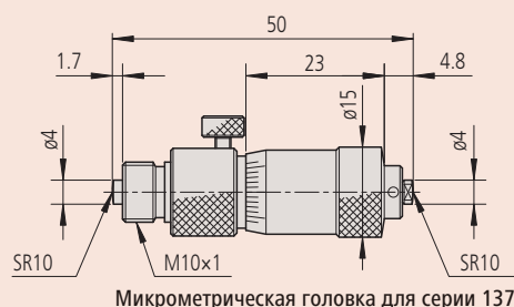
Микрометрическая головка для серии 137
