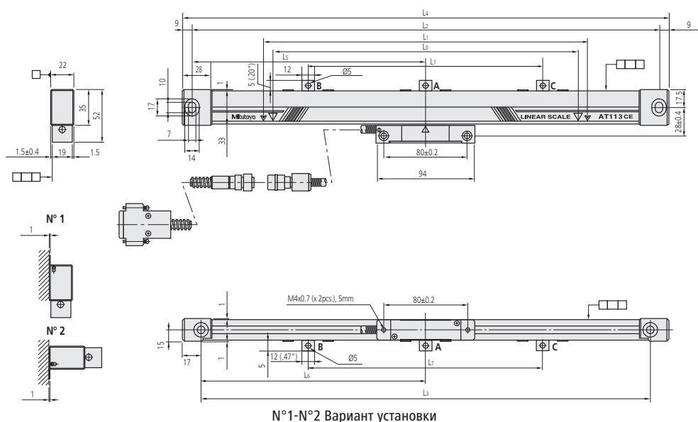
№1-№2 Вариант установки
