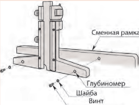
Установка сменного основания
