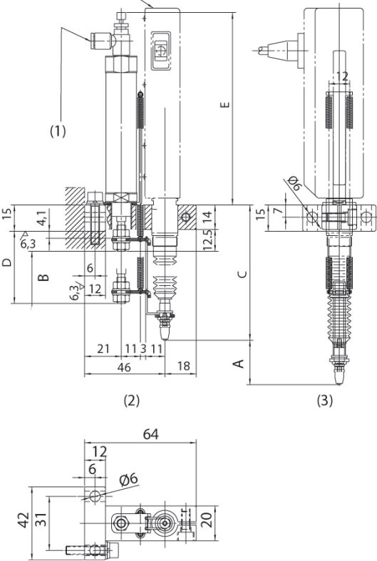
Для датчиков линейных перемещений с диапазоном 25 мм и 50 мм 1. Контроллер скорости 2. При выключенной подаче воздуха 3. При включенной подаче воздуха
