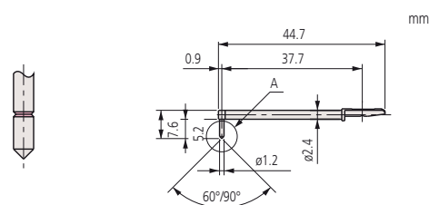
Стандартный щуп
