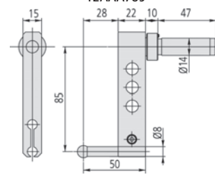
12AAA792 (с опциональным измерительным наконечником)
