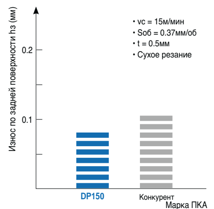
Обработка твердого сплава
