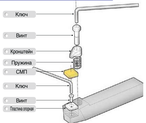
Прижим сверху. Тип С
