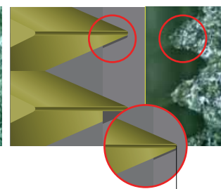
Резьба теряет форму из-за ошибки синхронизации
