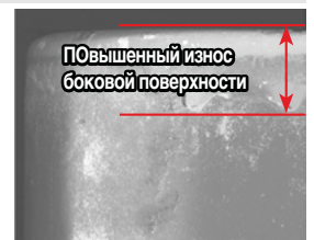
Существующие сплавы (K15)
