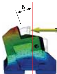
TBC460 (старый тип)
