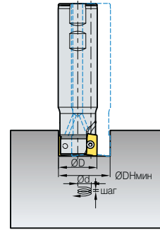
3. Винтовое врезание для сквозных отверстий
