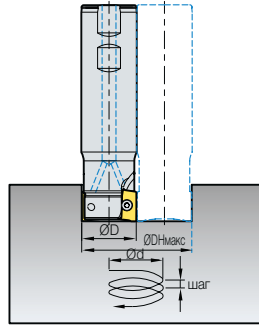
2. Винтовое врезание для глухих отверстий
